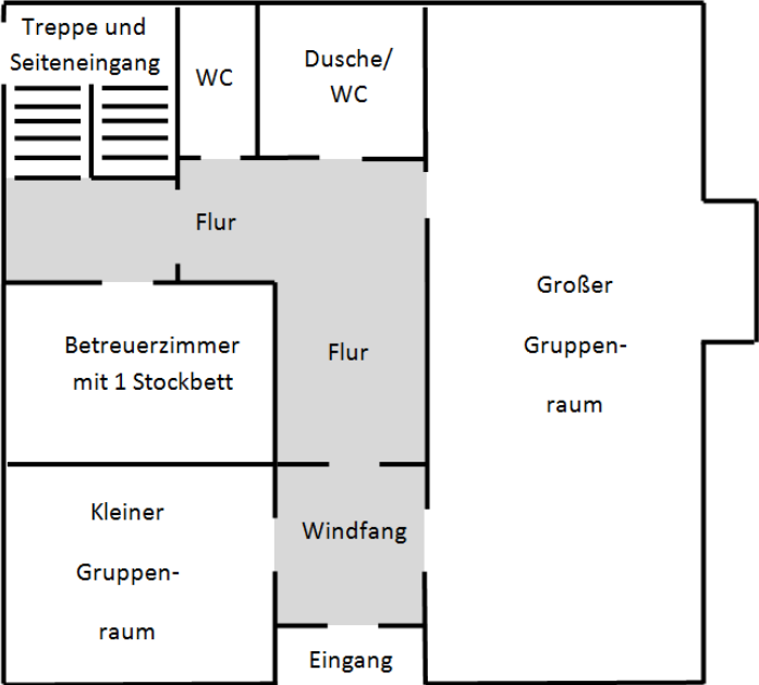
Erdgeschoss
